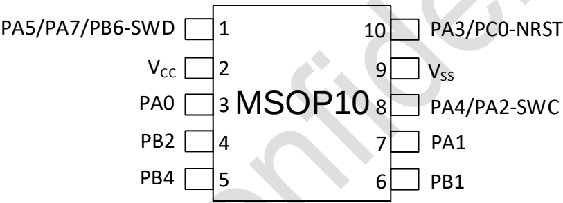
图 3-2 MSOP10 Pinout2 PY32M010A25N7
