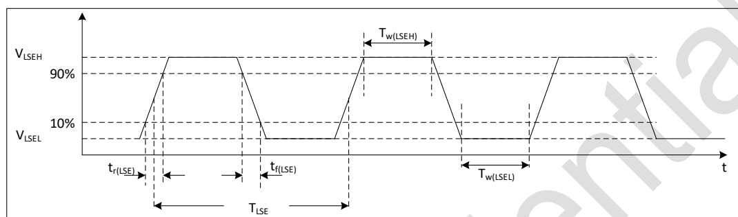
图 5-1 外部低速时钟时序图
